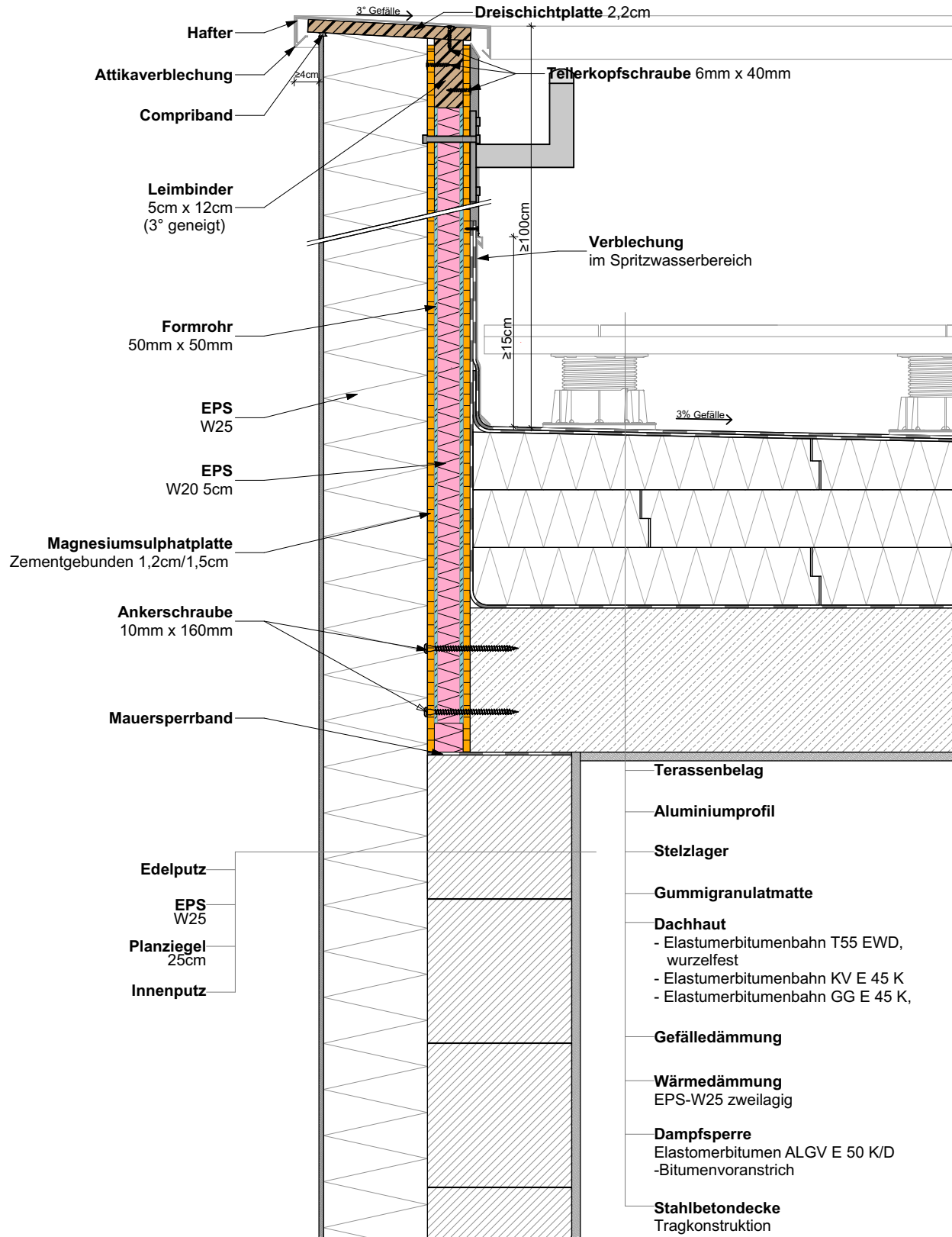
Brüstungssystem AS Schörflinger 25 MB - M 1:10 (Eigene Darstellung)
